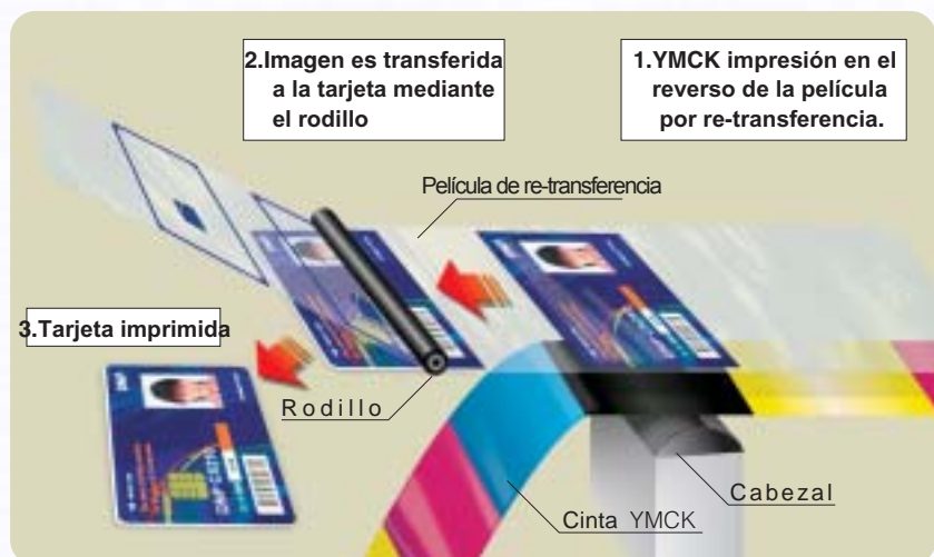
Proceso de impresión por re-transferencia ( explicación ilustrativa )
